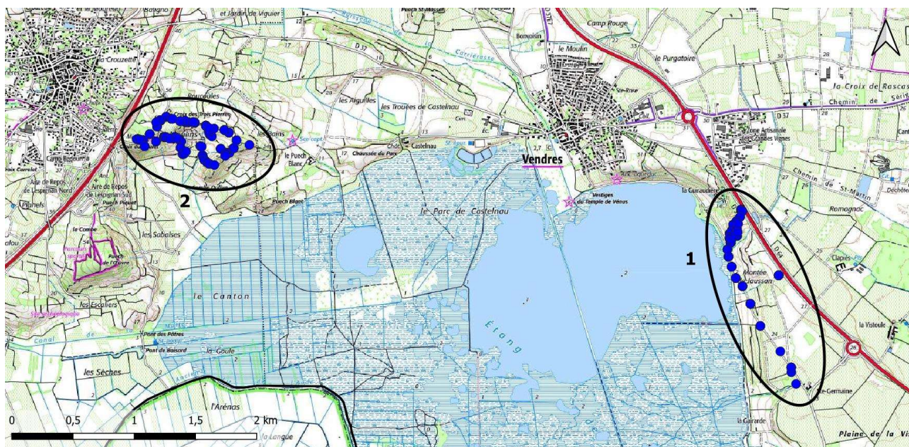
Carte 1 : Carte topographique avec les zones d'herborisation (source : https://www.geoportail.gouv.fr/ )
