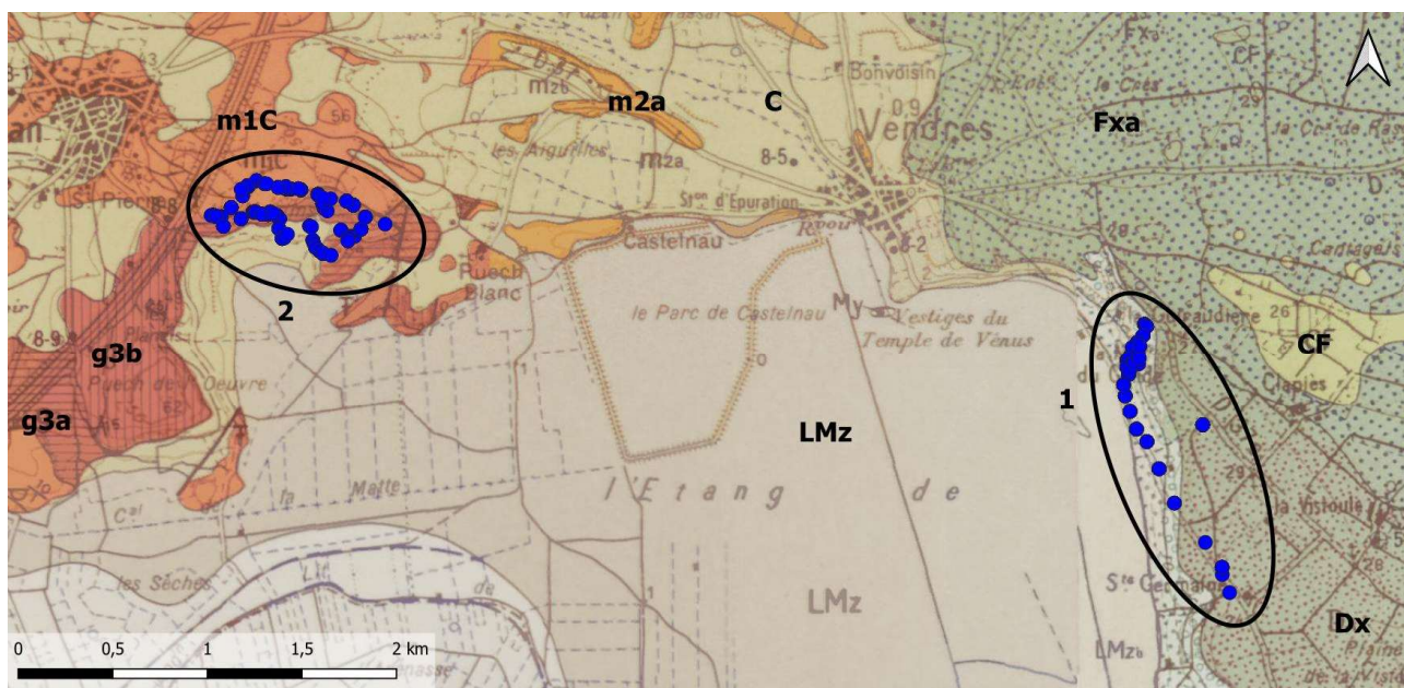
Carte 2 : Carte géologique avec les zones d'herborisation (source : http://infoterre.brgm.fr/ )
